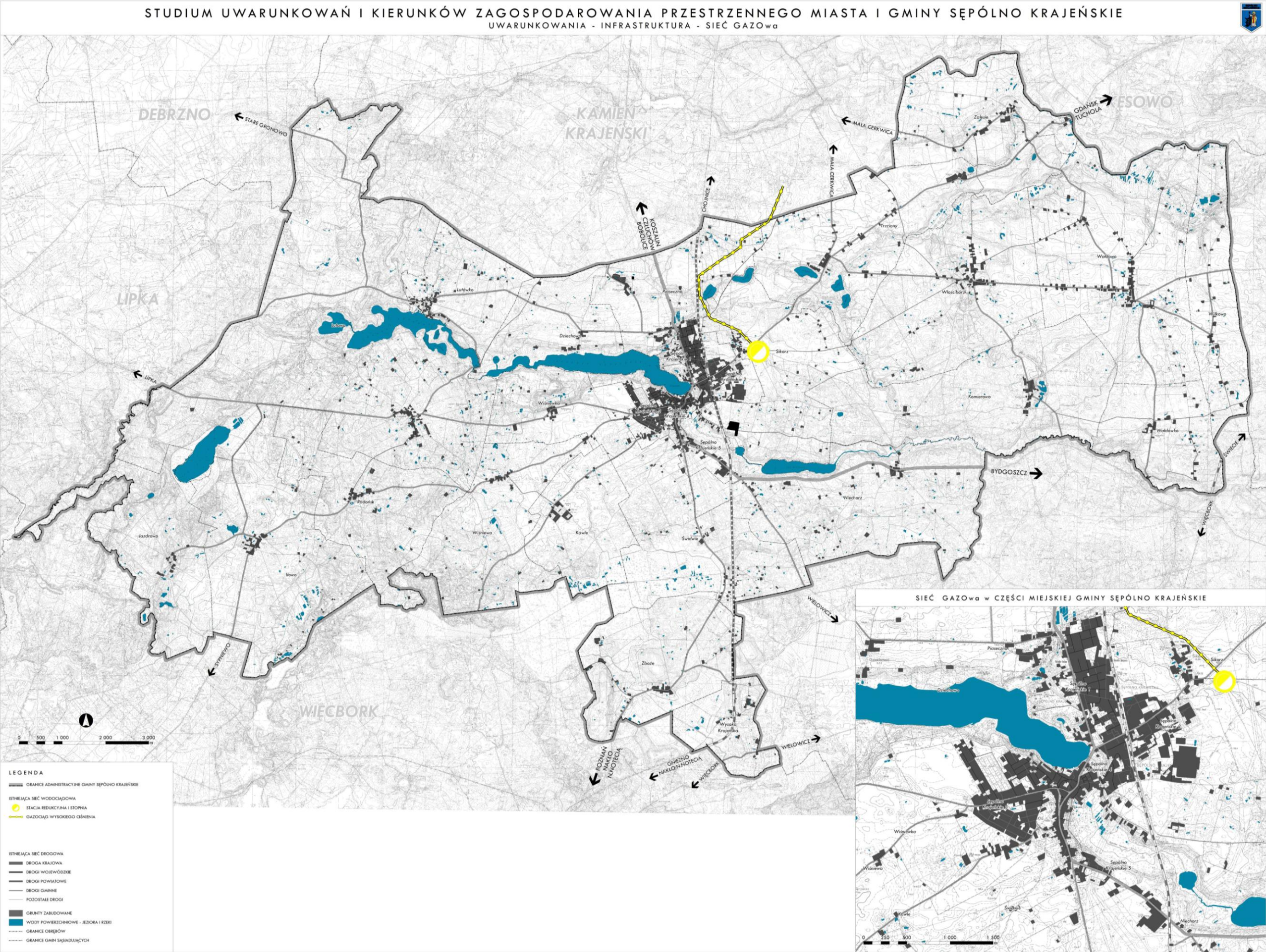
Rysunek 14. Sieć gazowa w gminie, opracowanie własne.
